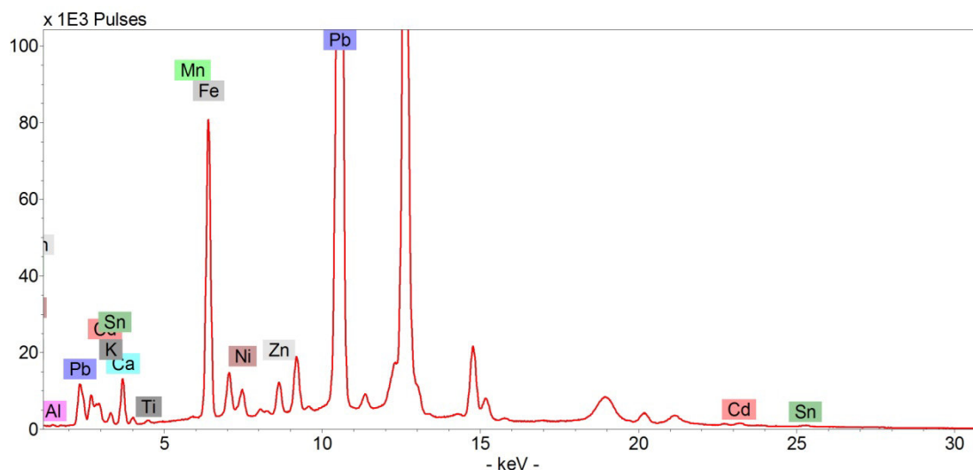
Figura 20. Espectro p-XRF de la muestra LPC-215-19 (Archivo fotográfico CNCR. Analista: T. Aguayo, 2018).
