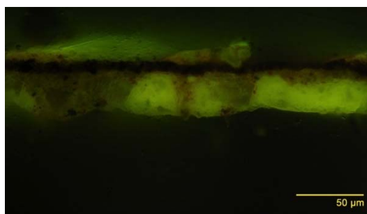
Figura 6. Microfotografía de la muestra LPC-156-06, bajo luz polarizada incidente (izq.) y bajo luz UV (der.).
