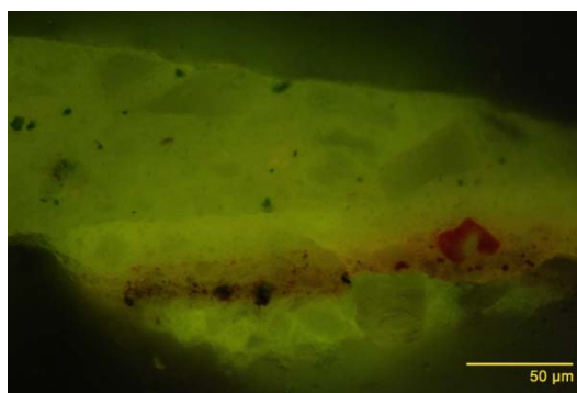
Figura 8. Microfotografía de la muestra LPC-156-08, bajo luz polarizada incidente (izq.) y bajo luz UV (der.).
