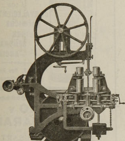
Fig. 5025. Sierra huincha con rodillos
