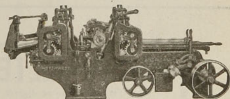
Fig. 679. Acepilladora y machihembradora
